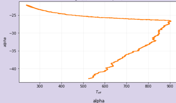
walking T_{eff} : 525.7 & \alpha_0 : -42.8
